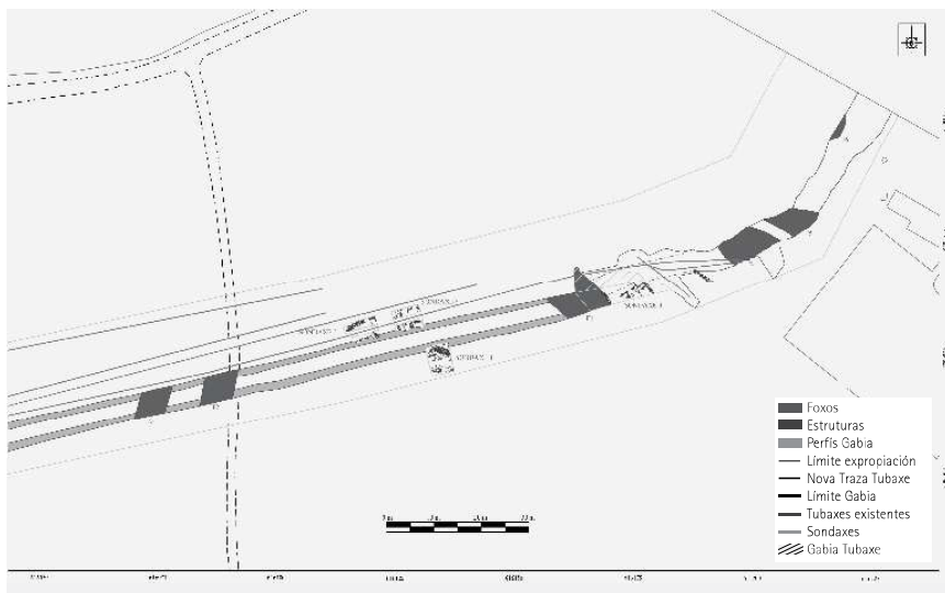
7. Planimetría da intervención
